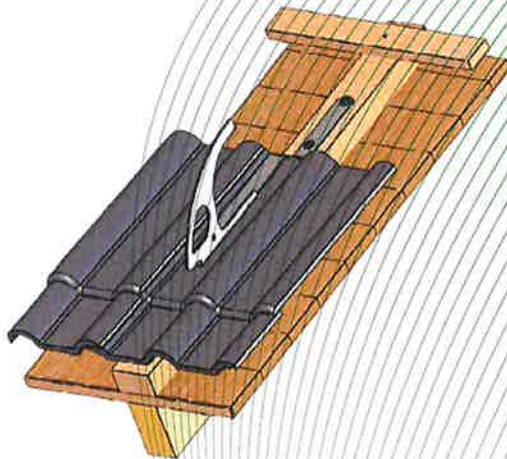
Bild 1: Sicherheitsdachhaken, Typ: GRH04
